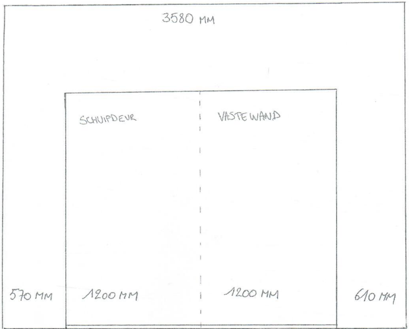
VOORAANZICHT
