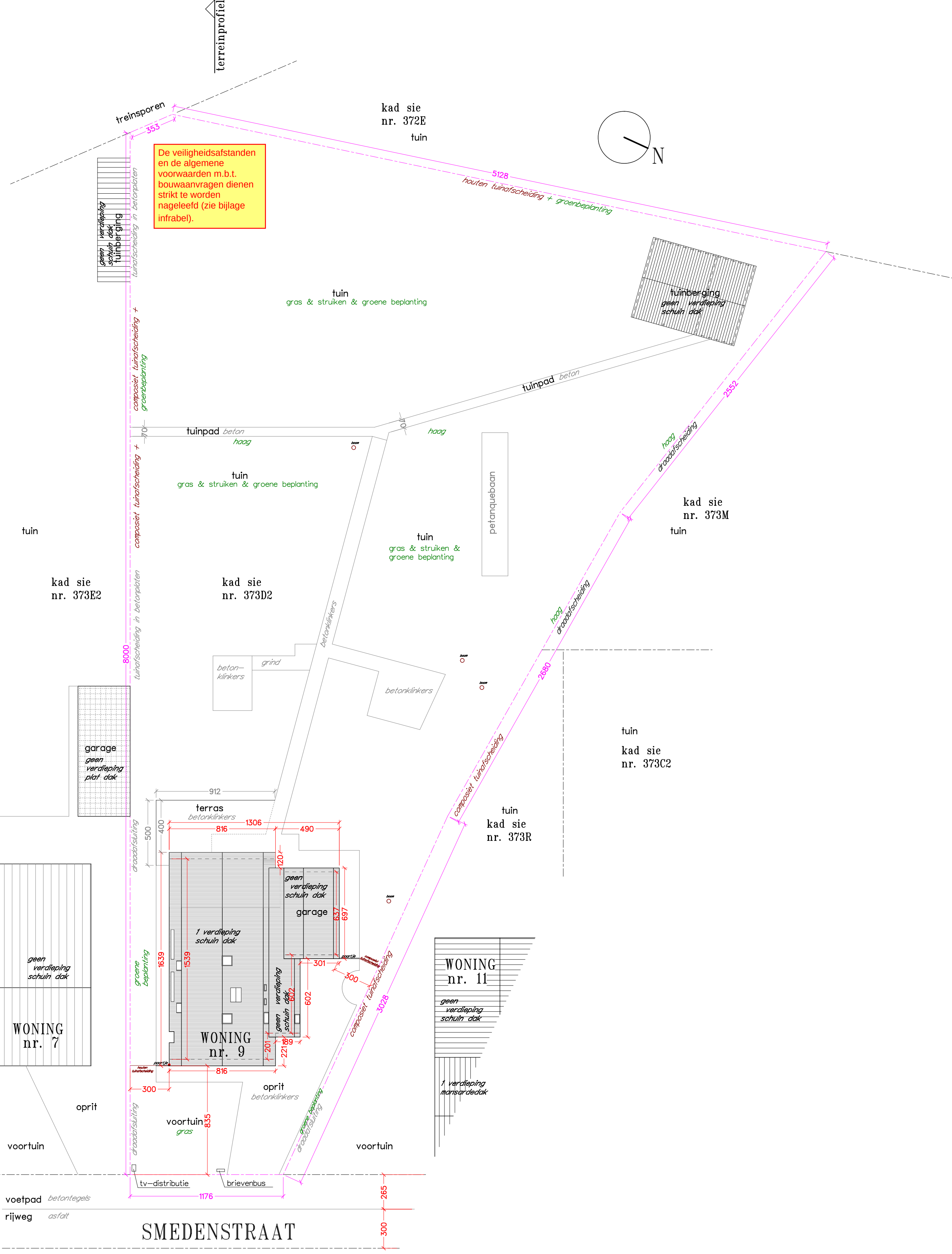
INPLANTINGSPLAN (nieuwe toestand) schaal 1/200 afmetingen in cm 0 400
